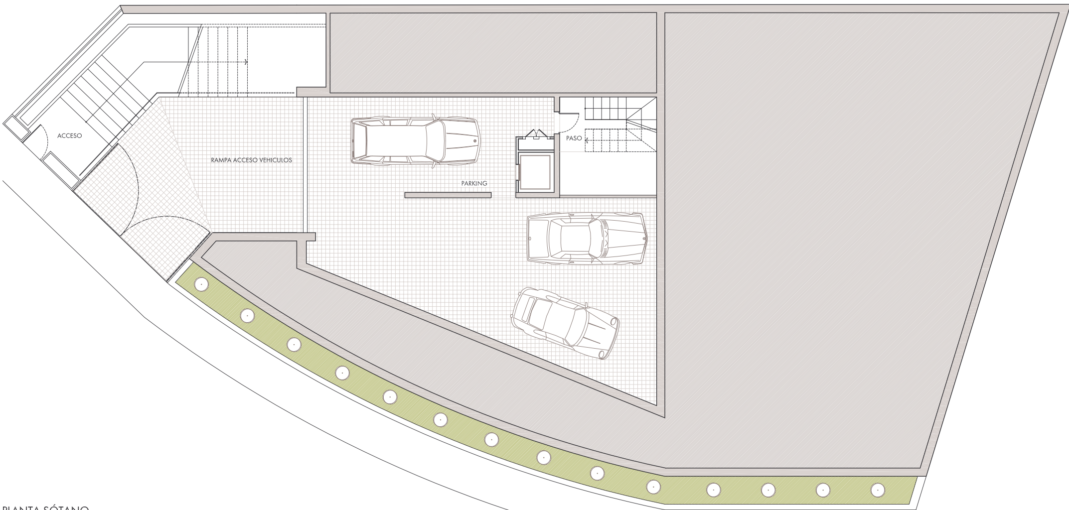
PLANTA SÓTANO
